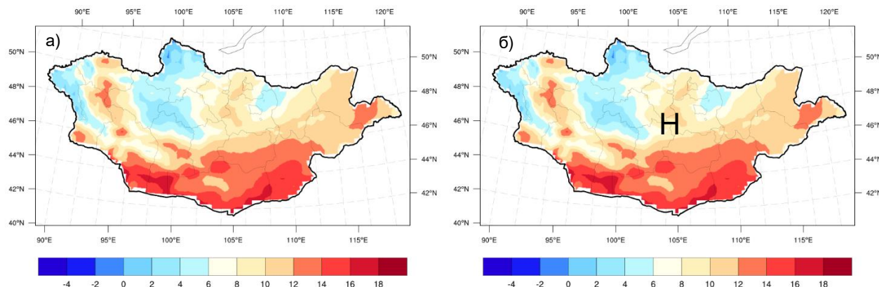
Зураг 3а. 9 дүгээр сарын агаарын температурын ОЖД (1991-2020)
