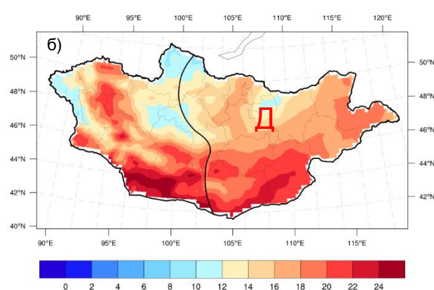
Зураг 1б. 8 дугаар сарын агаарын температурын урьдчилсан төлөв (°C)
