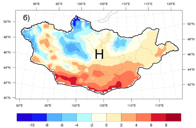
Зураг 3б. 10 дугаар сарын агаарын температурын урьдчилсан төлөв ( ^{\circ}\text{C} ) [Н – агаарын температур ОЖД-ийн орчим]
