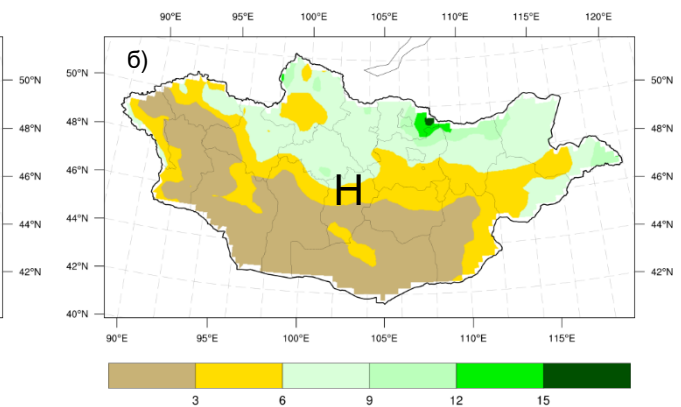
Зураг 6б. 10 дугаар сарын хур тунадасны урьдчилсан төлөв (мм) [Н-хур тунадас ОЖД-ийн орчим]
