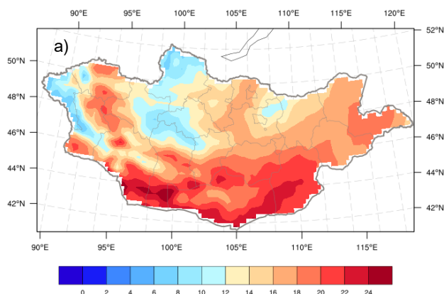
Зураг 1а. 8 дугаар сарын агаарын температурын ОЖД (1991-2020)
