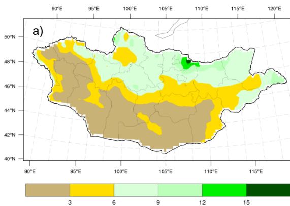
Зураг 6а. 10 дугаар сарын хур тунадасны ОЖД (1991-2020)
