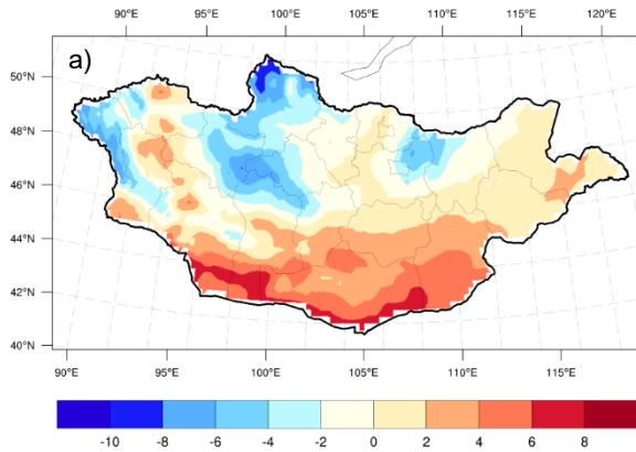
Зураг 3а. 10 дугаар сарын агаарын температурын ОЖД (1991-2020)
