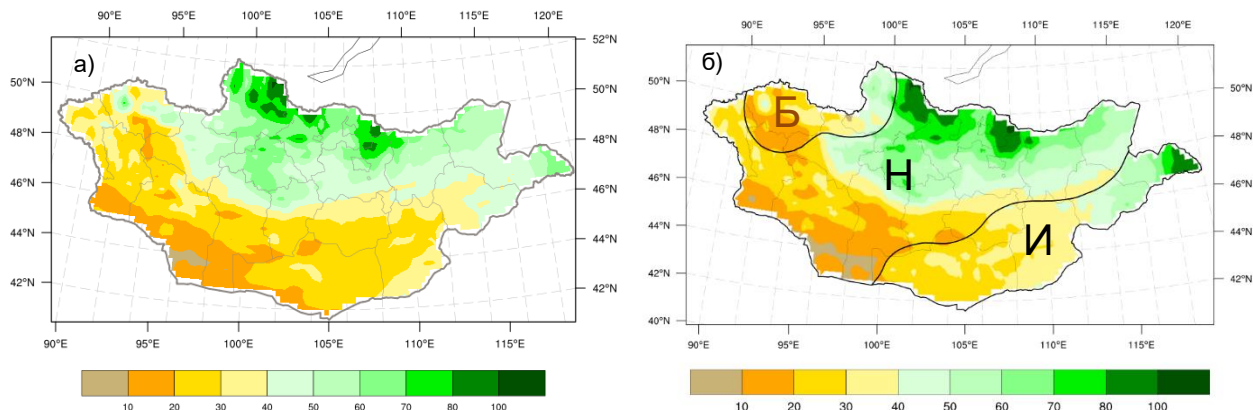
Зураг 2а. 8 дугаар сарын хур тунадасны ОЖД (1991-2020)
